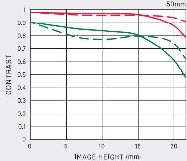
波動光学的MTF
